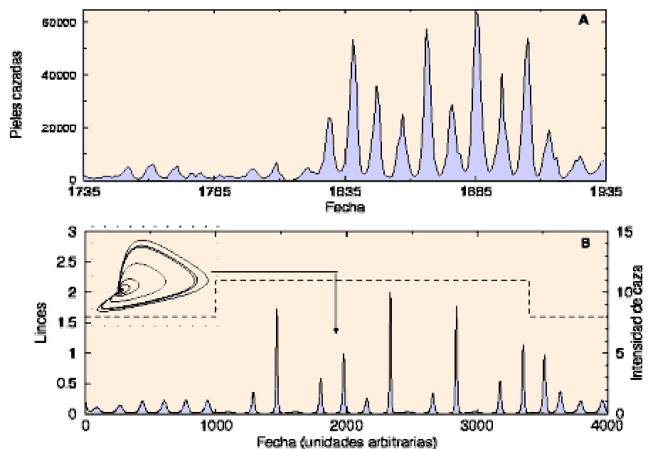
Figura 1. (A) Serie de pieles de linco cazadas durante dos siglos. (B) Serie simulada (línea continua) con cambios bruscos en la presión de caza (línea discontinua). Con alta presión de caza la serie describe un atractor extraño.
