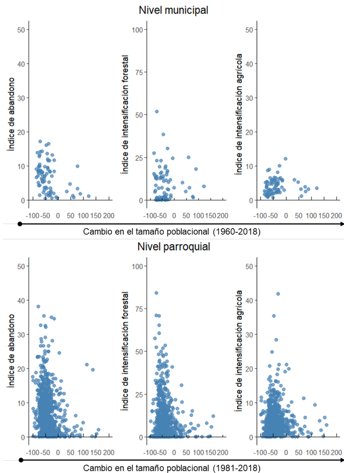
Figura A1. Representación mediante nube de puntos de los valores de los índices de abandono e intensificación de usos del suelo para cada nivel de análisis (municipio y parroquia).
