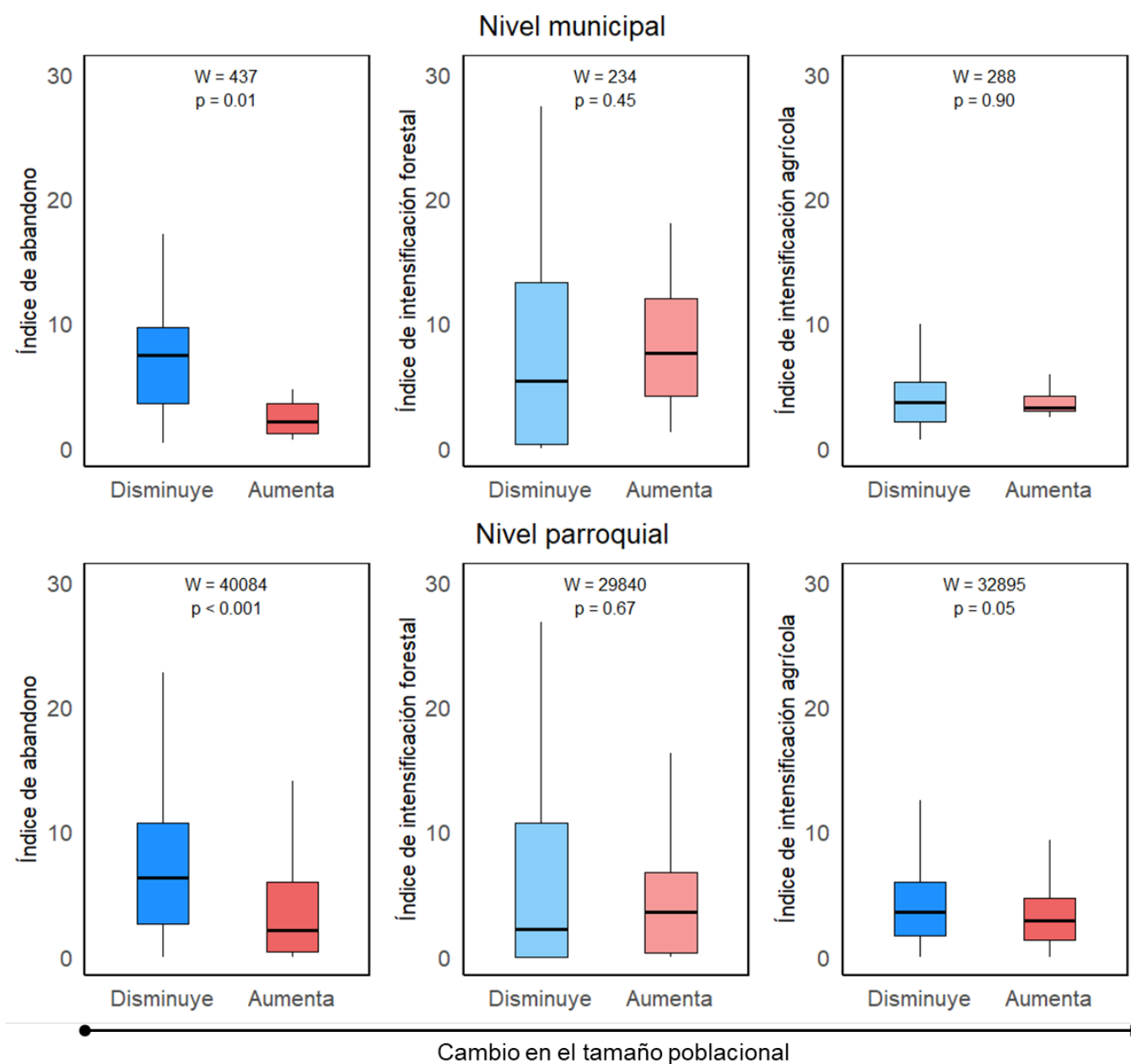
Figura 4. Diagramas de cajas que representan los valores de los índices de abandono e intensificación de usos para las unidades administrativas consideradas (municipios y parroquias), clasificadas según su dinámica demográfica: disminución (azul) o aumento (rojo) de la población. Se incluyen los resultados de la prueba U de Mann Whitney (W) aplicada a cada índice y nivel de análisis. Las diferencias estadísticamente significativas se destacan con tonos de color más intensos.
