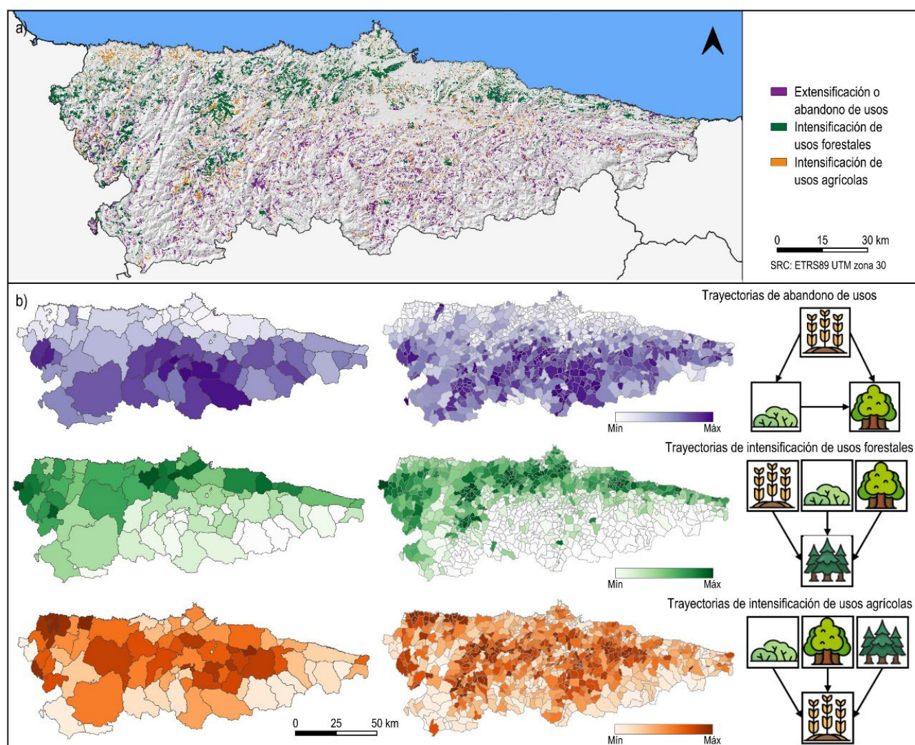
Figura 3. a) Distribución de las zonas afectadas por abandono (morado), intensificación forestal (verde) e intensificación agrícola (naranja). b) Distribución a nivel municipal (izquierda) y a nivel parroquial (derecha) del valor promedio por unidad administrativa de los índices de abandono (morado), de intensificación forestal (verde) y de intensificación agrícola (naranja).
