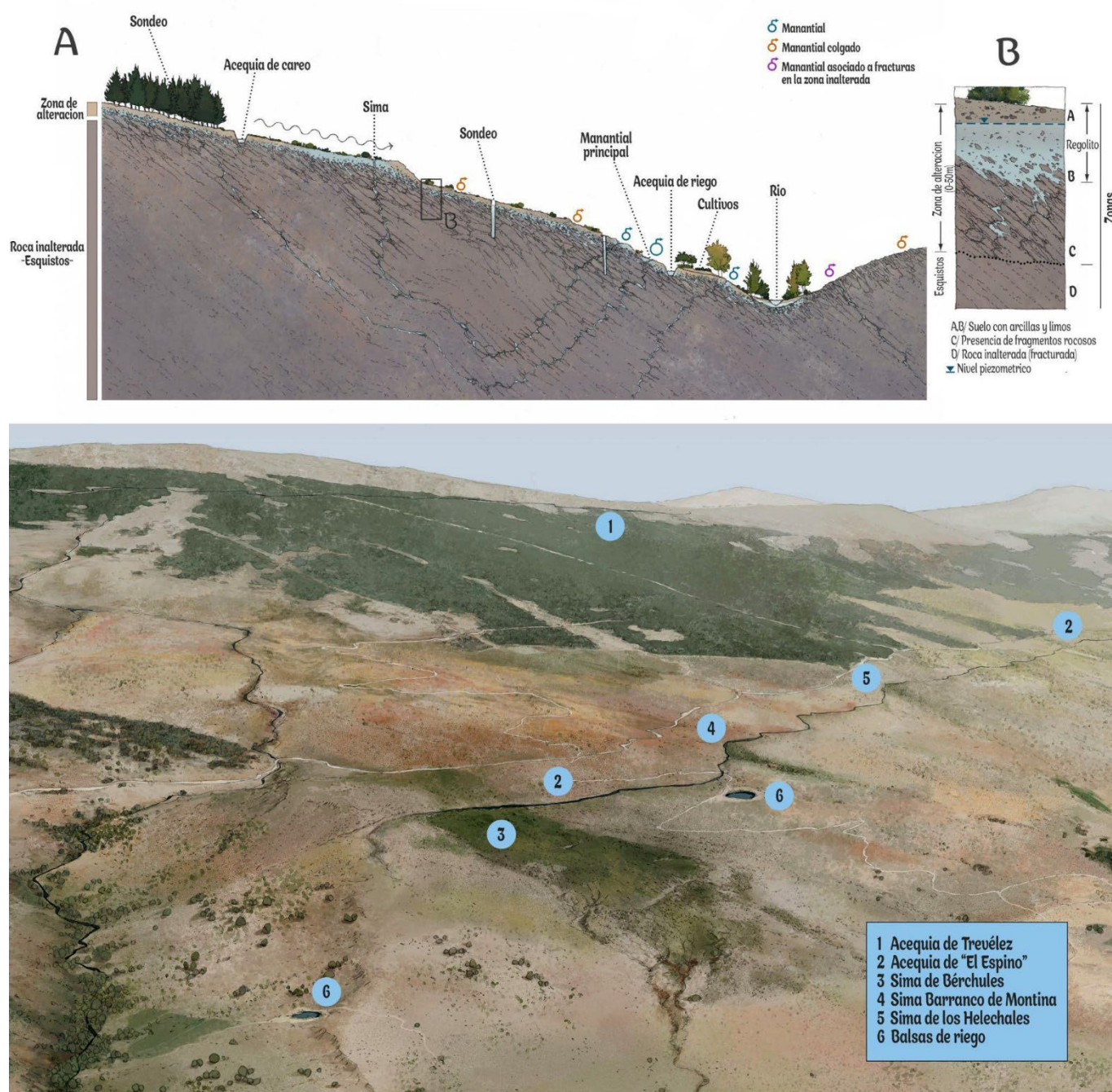
Figura 2. Acequias tradicionales y funcionamiento hidrogeológico de laderas en Sierra Nevada. Arriba A: Esquema de funcionamiento hidrogeológico en una ladera de Sierra Nevada donde las acequias de careo y de riego, y los retornos de los riegos por inundación recargan a los acuíferos en pendiente. Arriba B: Detalle de la zona de alteración de los afloramientos de esquistos por la que circula el agua subterránea. Los esquistos inalterados (D) funcionan como base de baja permeabilidad de estos acuíferos. Debajo: Panorámica del tramo final de la acequia de careo del Espino, en la cuenca del río Bérchules. Se observan varias "simas" en las que se vierte el agua para su infiltración y en las que se generan pastos que destacan por su mayor verdor (Autora: Rocío Espín-Piñar).
